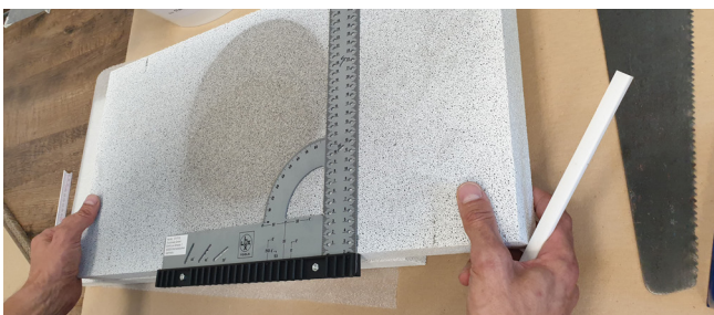
7. Für notwendige Zuschnitte, Gesamtbild beachten
